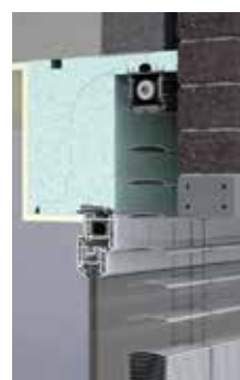
Ausführung Klinker
