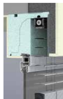
Ausführung WDVS
